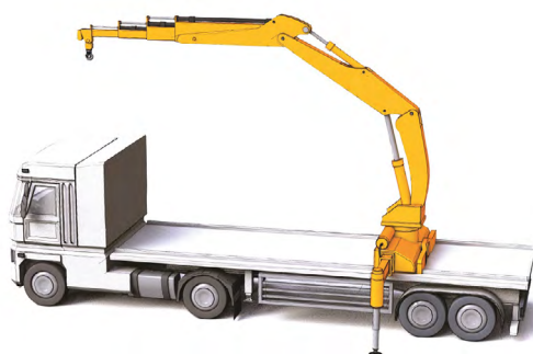
Grue de chargement montée en position centrale
